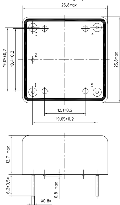
паяный корпус
